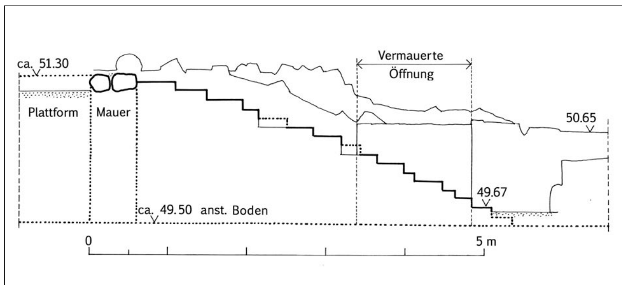
Abb. 18: Schematischer Längsschnitt durch Treppe 4. Auf 4,50 m Länge wird ein Höhenunterschied von 1,63 m überwunden. Aus diesem sehr bequemen Steigungsverhältnis ergeben sich 15 Stufen zu je 11 cm Höhe, mit 14 Auftrittsflächen von je 32 cm Breite. Die tatsächliche Ausführung ist jedoch sehr unregelmäßig und erfolgte sichtlich ohne entsprechende Planung (Zeichnung: D. Eigner).
