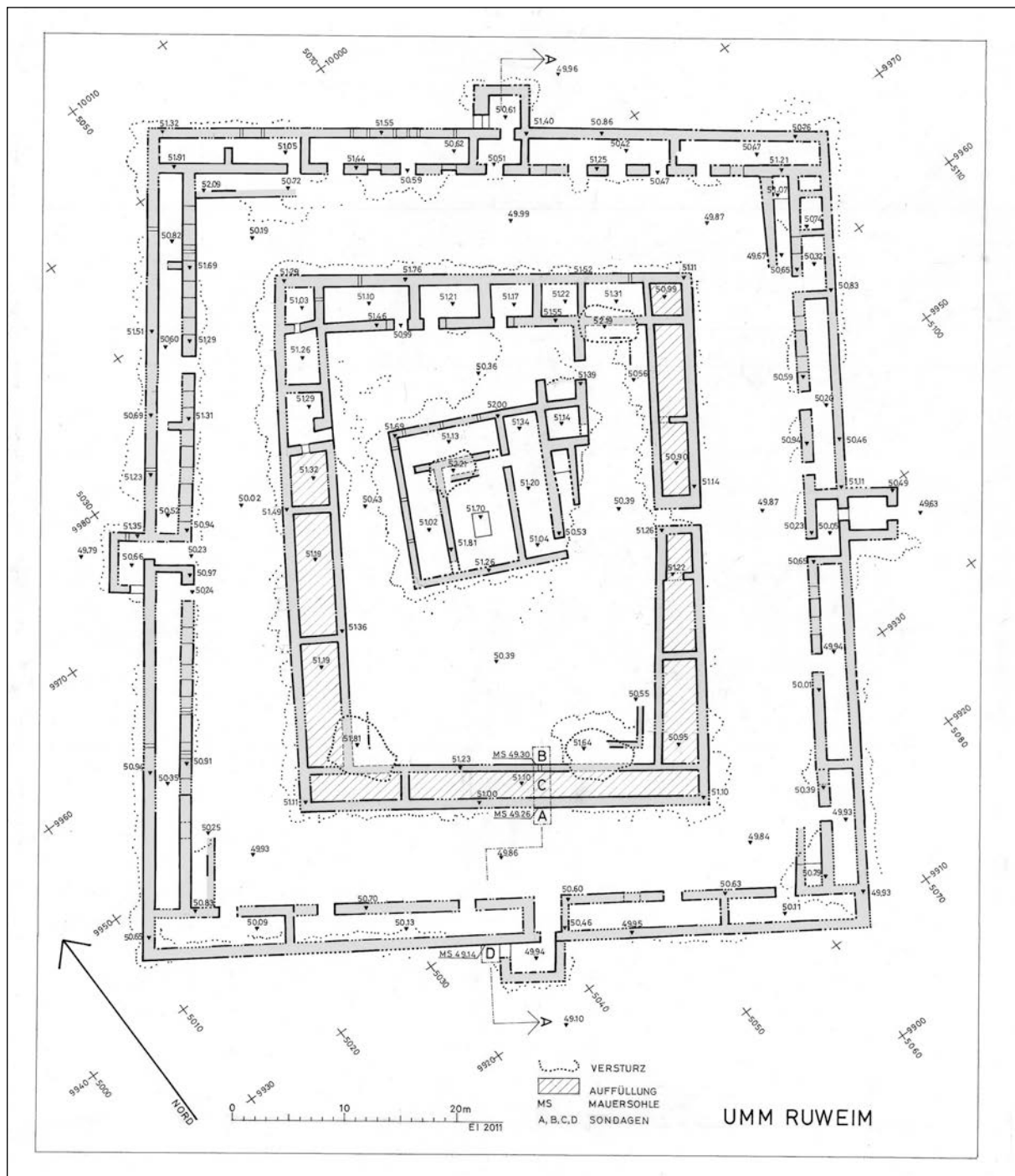
Abb. 4: Grundrissplan des Bauwerks Umm Ruweim 1 (Feldaufnahme D. Eigner & Tim Karberg, Zeichnung: D. Eigner).
